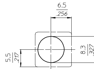
Einbaumaße Mounting layout
