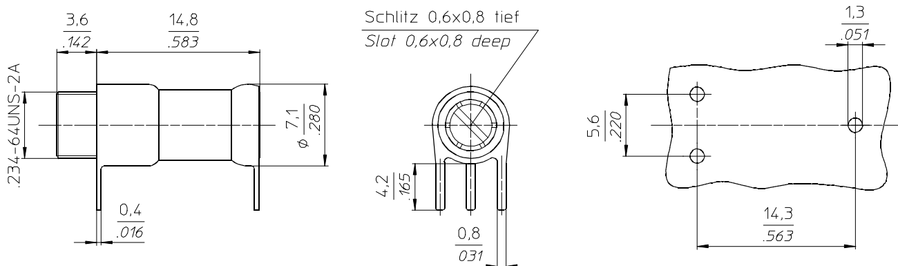
Einbaumaße Mounting layout
