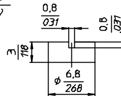
Dichtkappe geschlitzt lose Maß A +1,4 Slotted sealcap unmounted Dim A +.055
