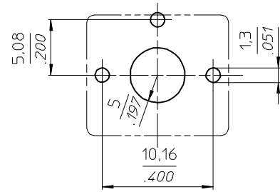
Einbaumaße Mounting layout
